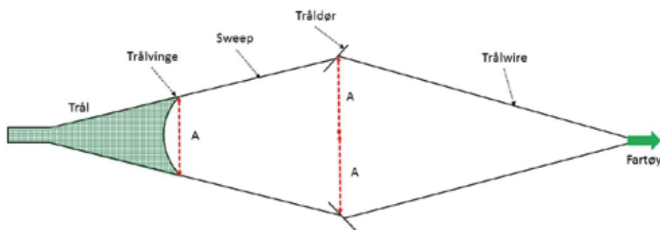
Figur 5: Hva er det egentlig som samler sammen fisken og hvor bredt fanger en pelagisk trål? Når WKWIDE forskerne får en mengdeindeks fra tråltoktet IESSNS som de mener er for stor, mener de at det er døravstanden ( 2x_A på figuren) som må brukes når de skal beregne tettheten av makrell i havet. Dette gir halve makrelltettheten og halve mengdeindeksen fra toktet i forhold til om de bruker avstanden mellom trålvengene (A). Ingen trålskipper vil være enige i at all fisken som passerer mellom tråldørene ender opp i trålen, og derved i trål-mengdeindeksen.
